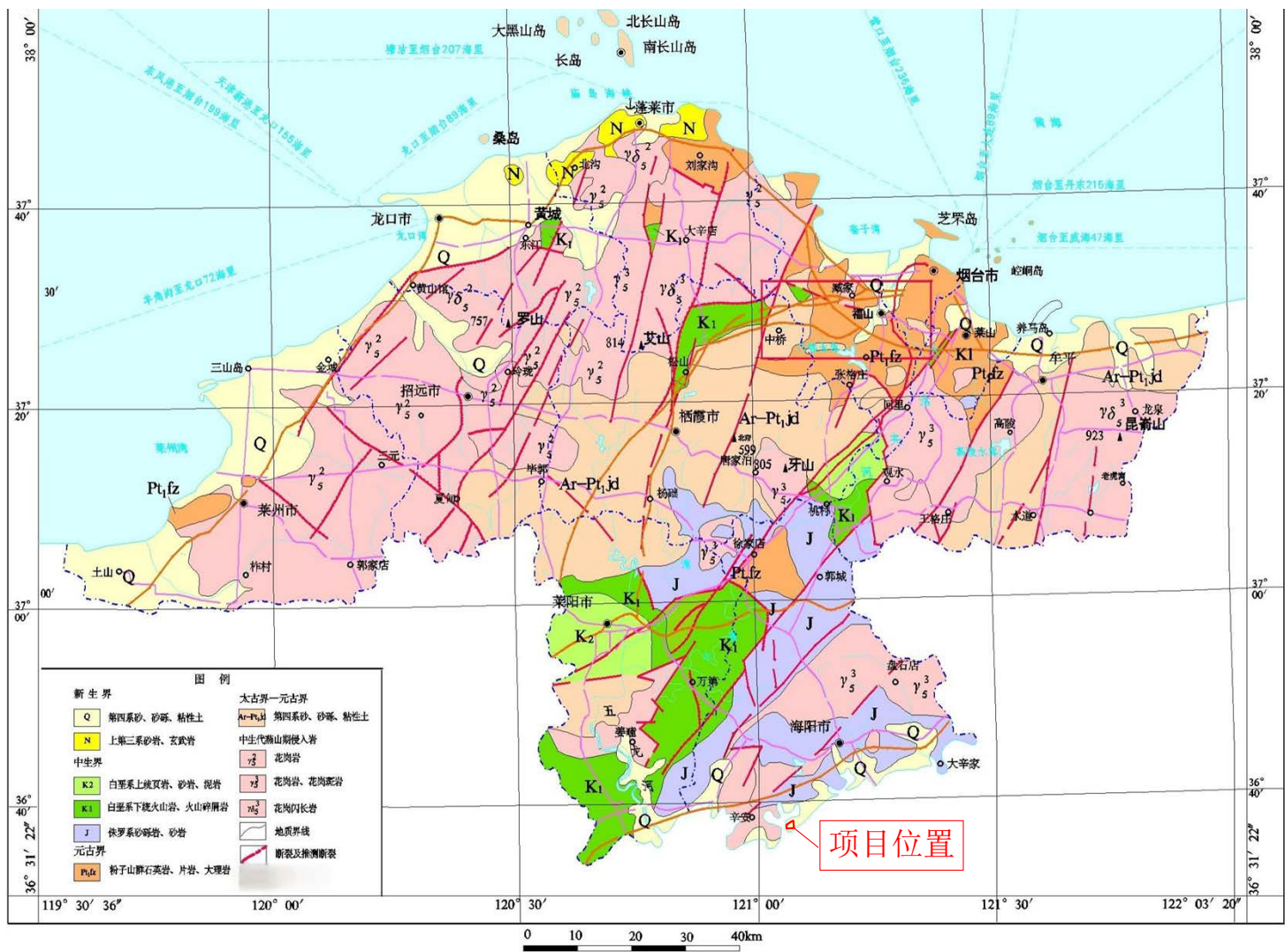
图 4.1-3 拟建项目所在区域地质构造图
