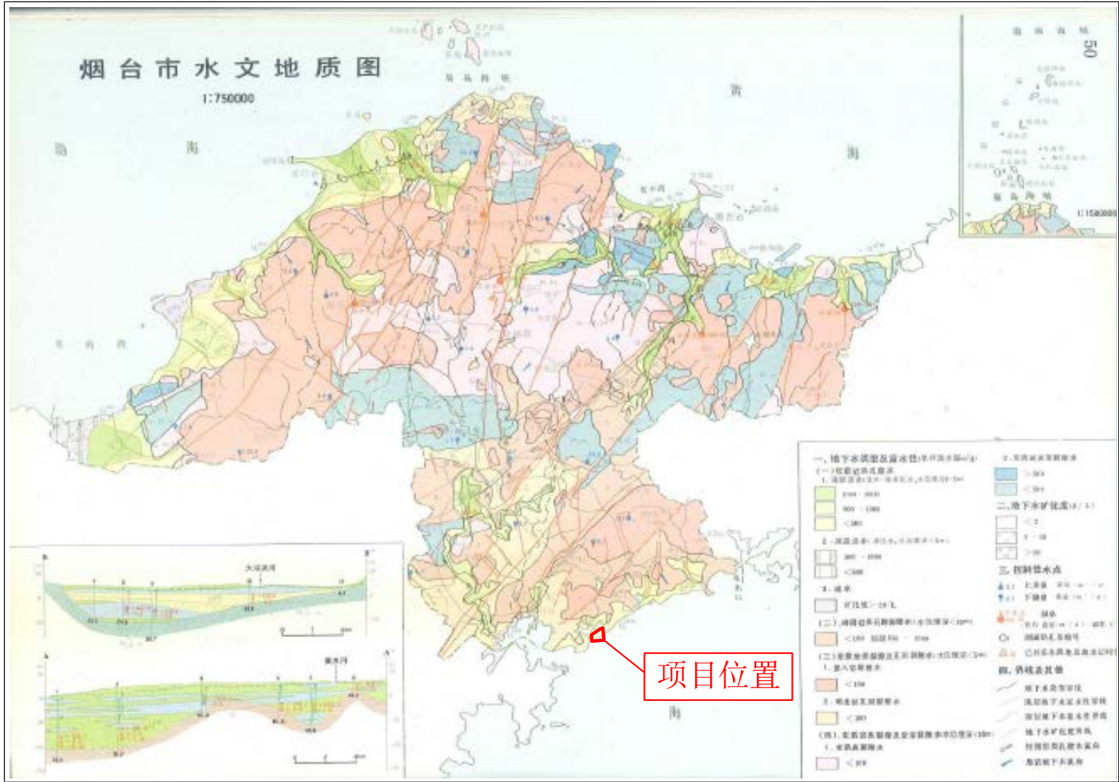
图 4.1-5 拟建项目所在区域水文地质图
