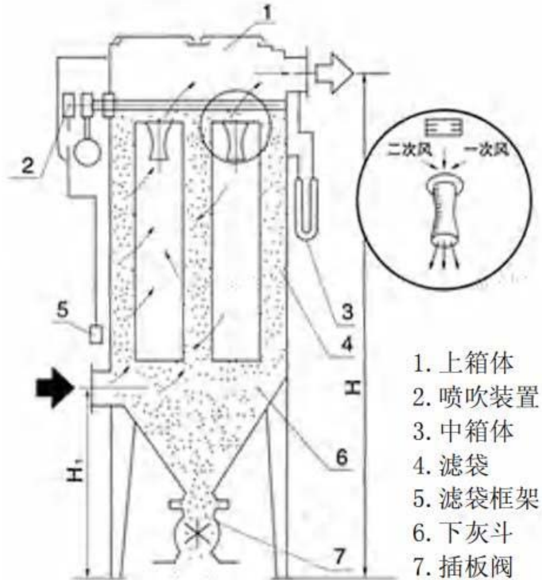
图 9.2-1 布袋除尘器结构图
